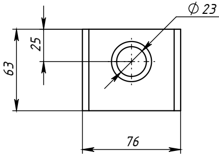
Поз.3 (Пластина) 1:3
