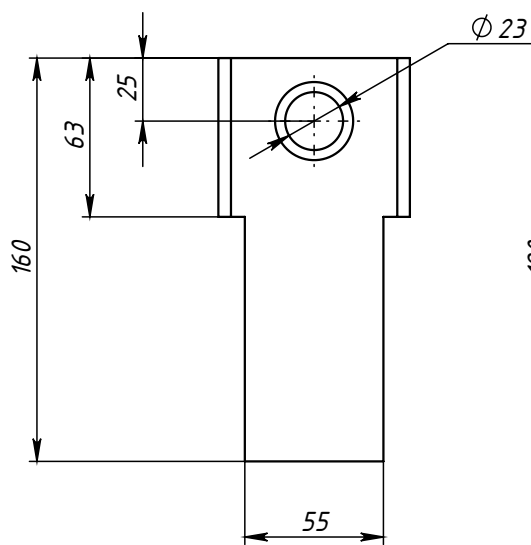
Поз.4 (Пластина) 1:3
